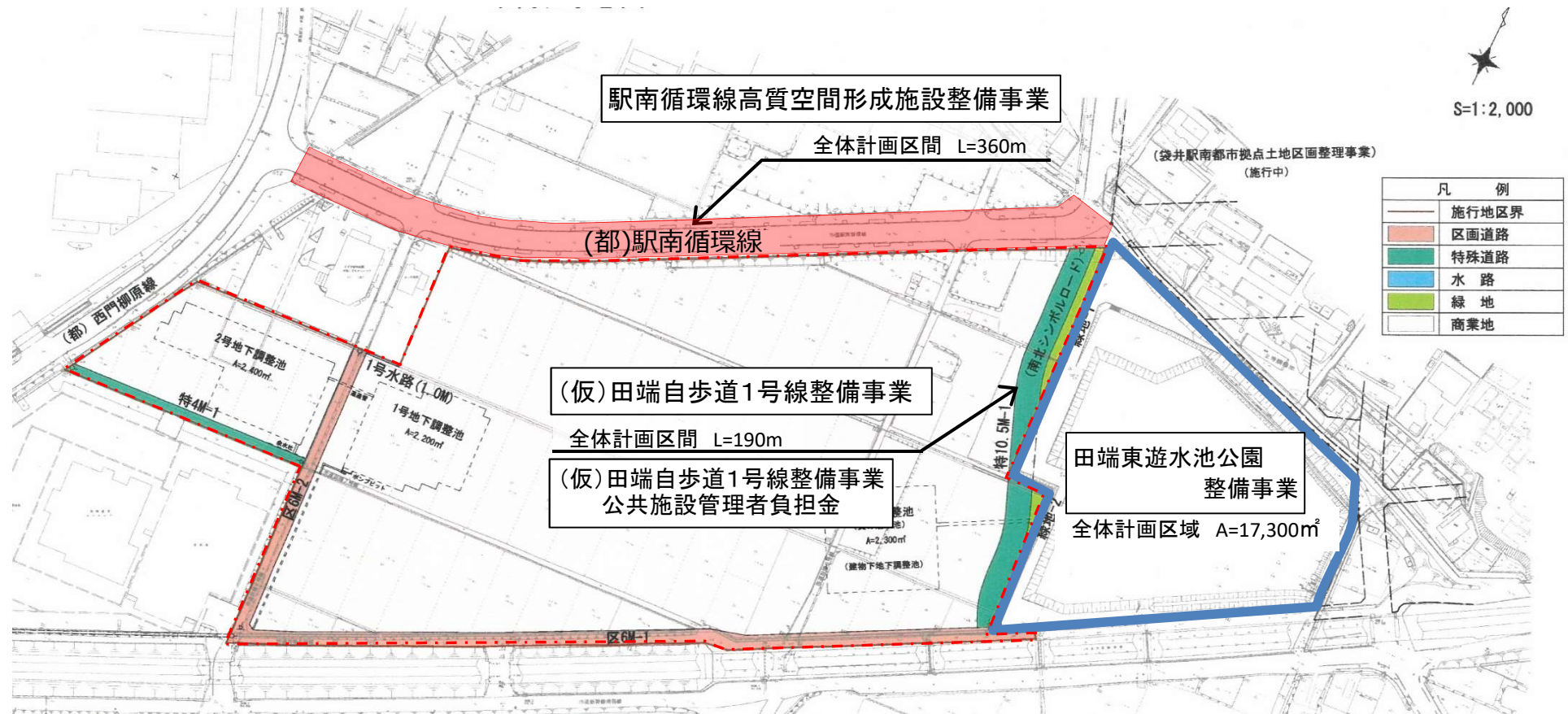
袋井駅南田端商業土地地区画整理事業 事業計画図
